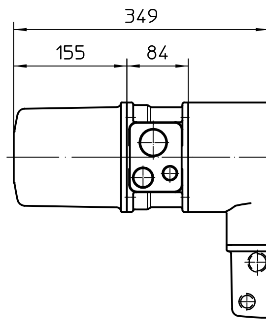
Ausführung mit therm. Überstromrelais
