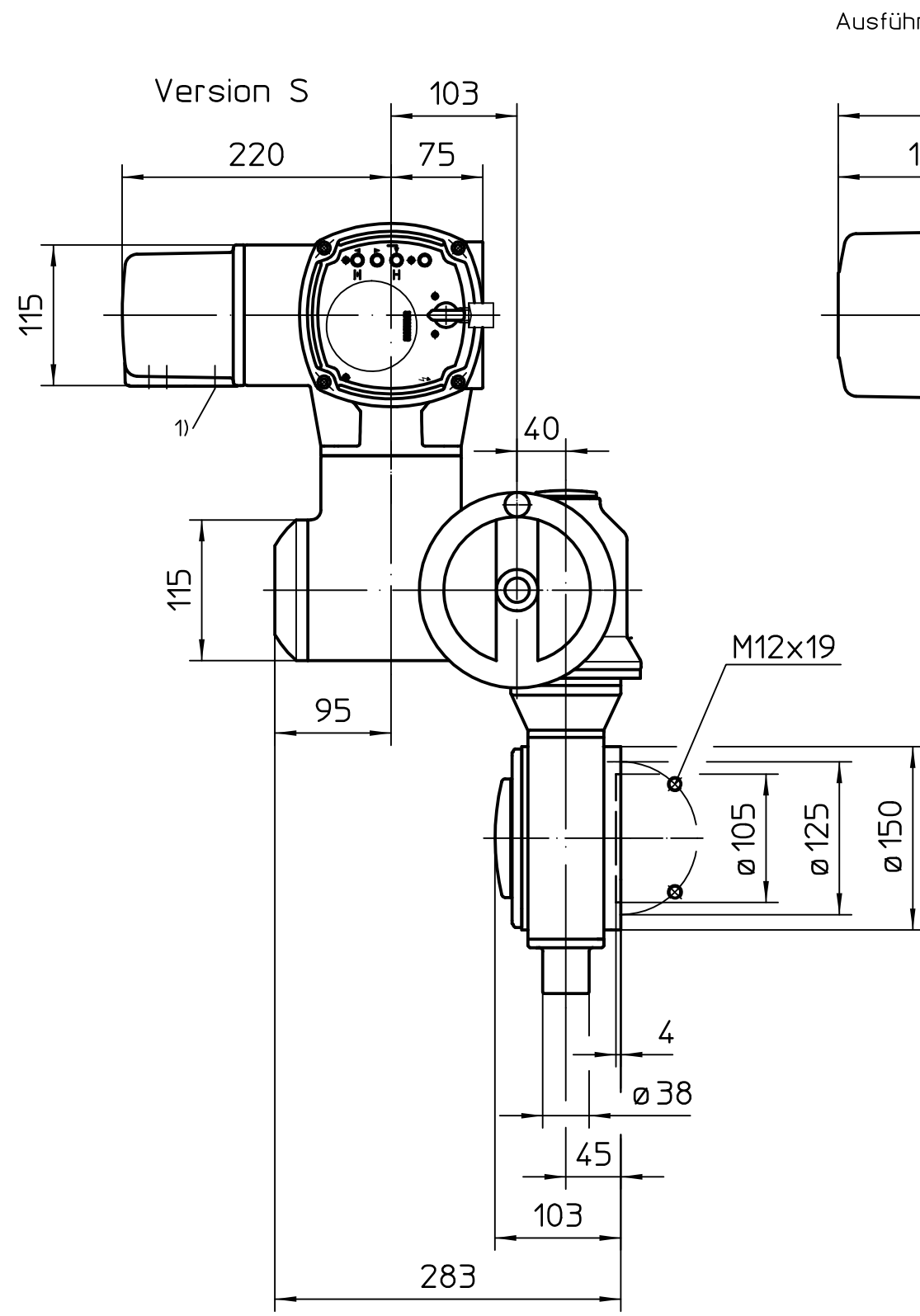
Ansicht A
