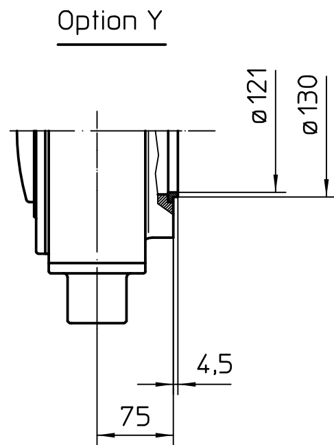
Ansicht A
