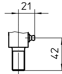
Detail X M 1:2,5
