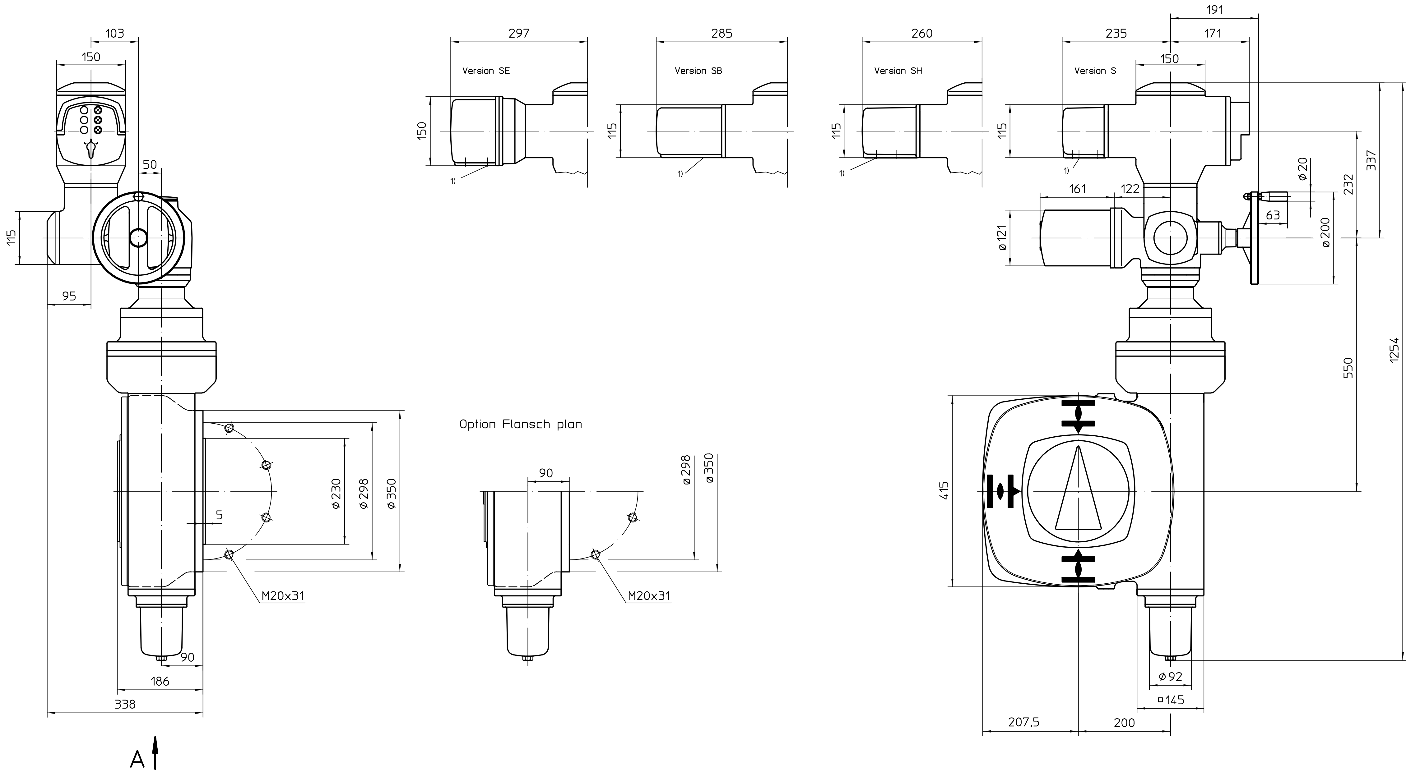
Ansicht A
