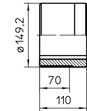
Kupplung
