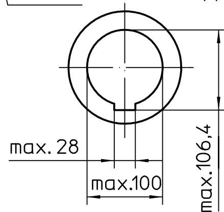
Kupplung
