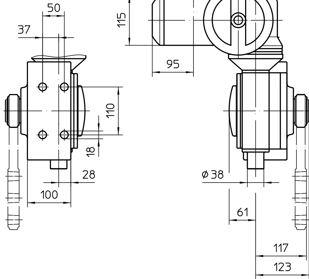
Ansicht A
