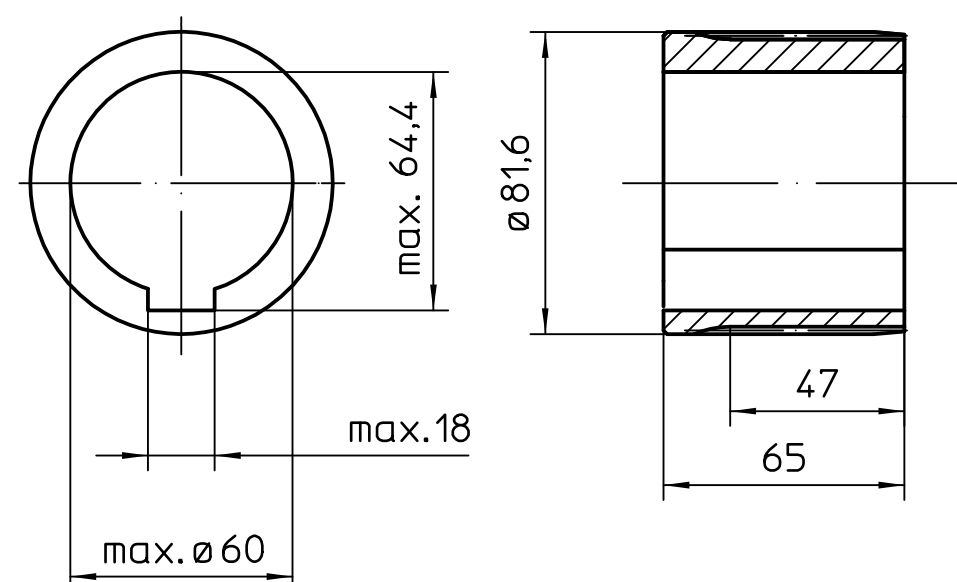
Kupplung
