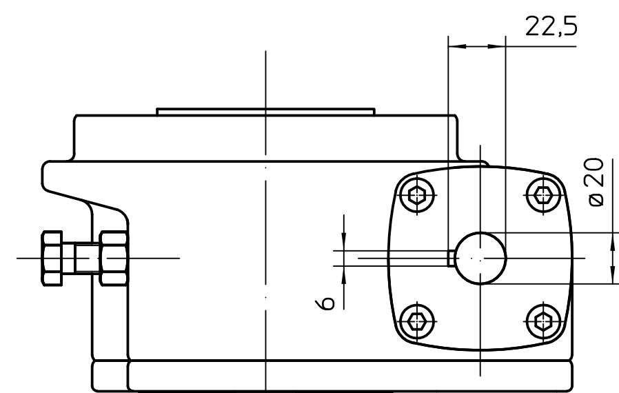
Kupplung
