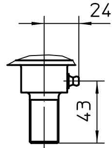
Detail X M 1:2,5
