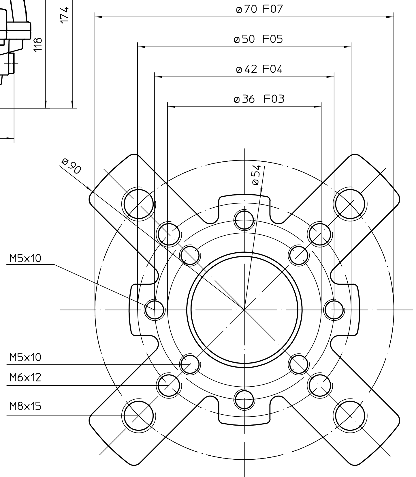
Ansicht A M 2:1
