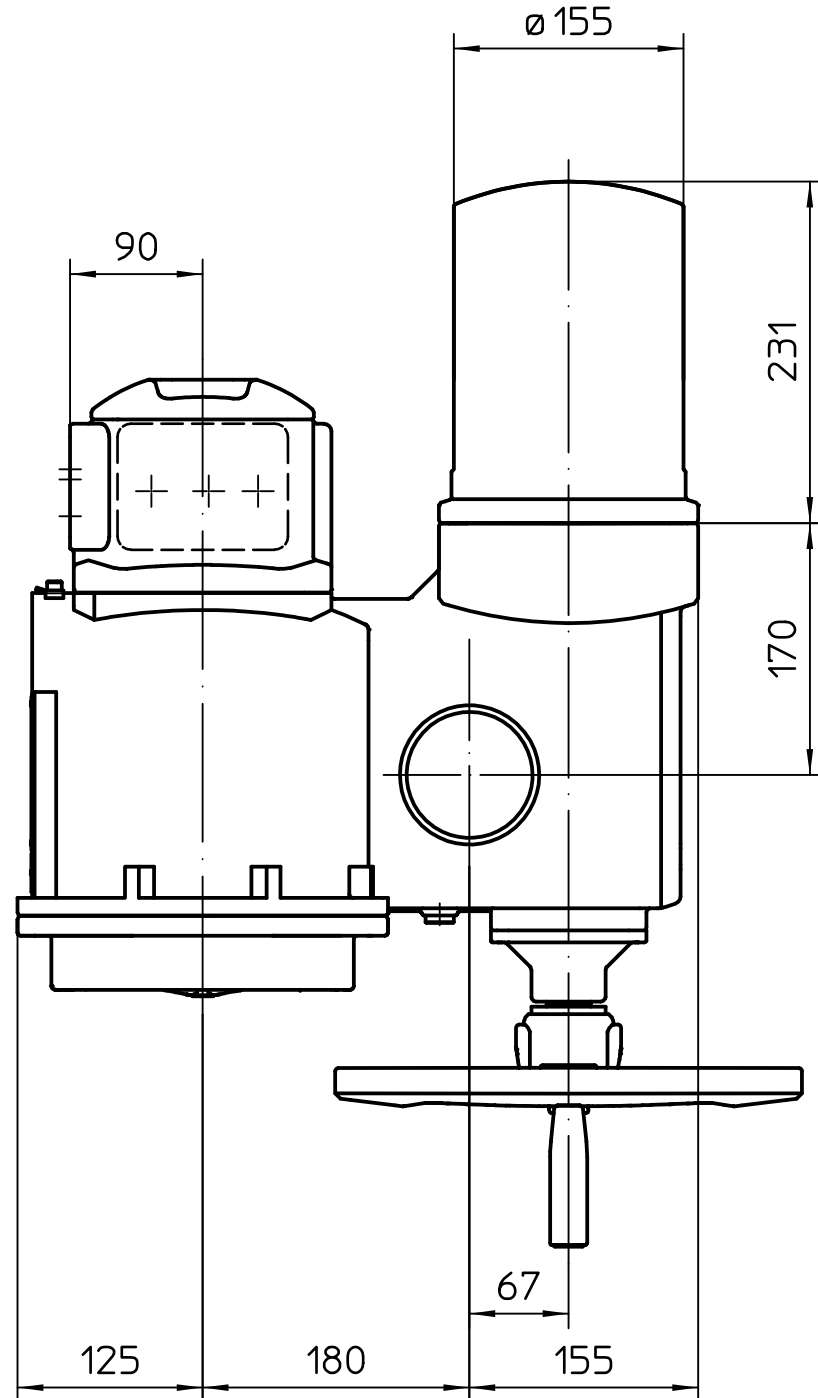
Ansicht A
