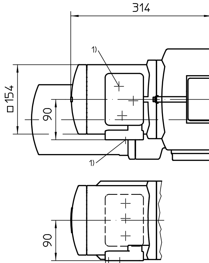
Ansicht A
