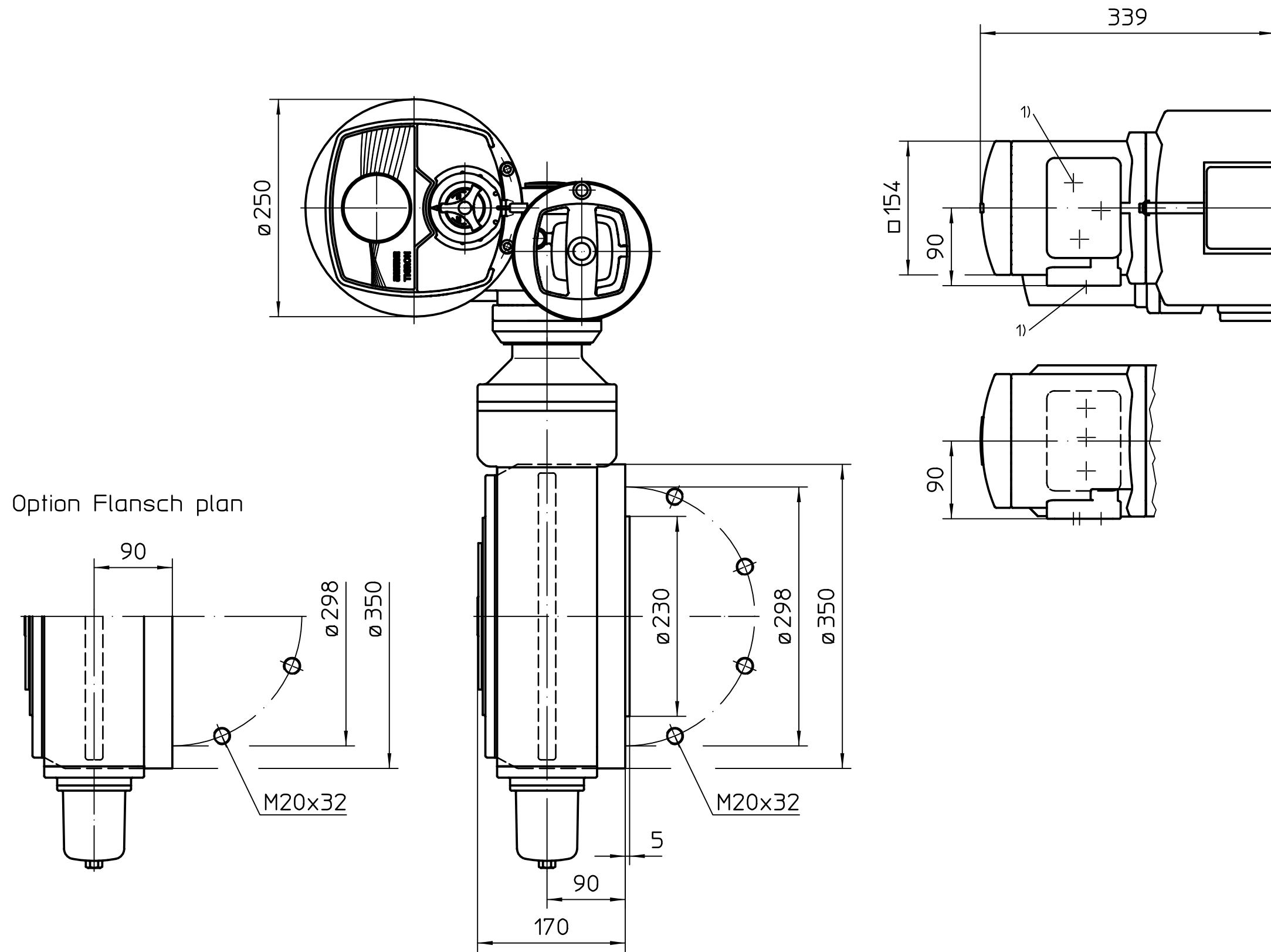
Ansicht A
