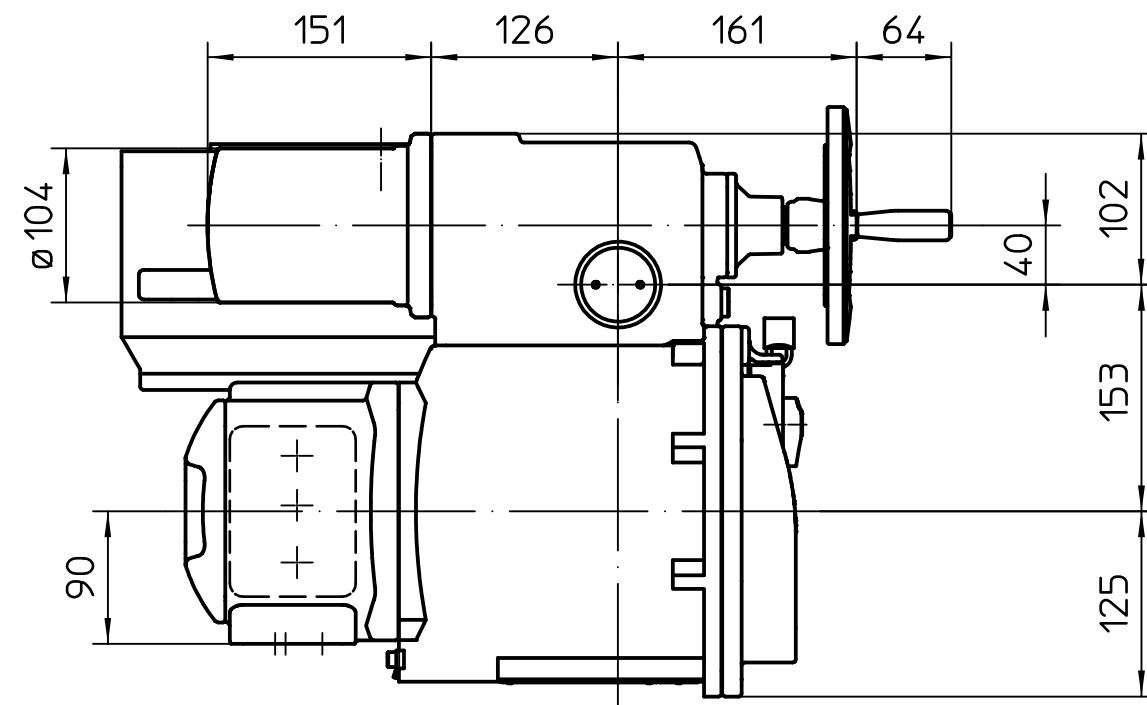
Ansicht A
