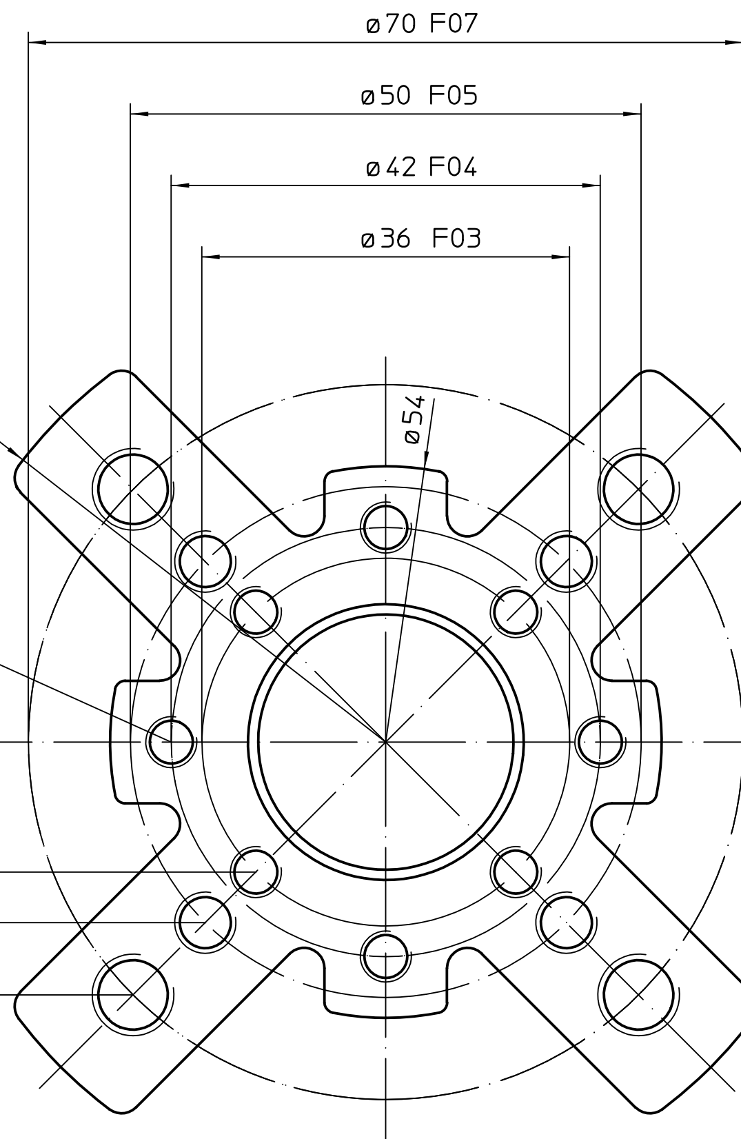
Ansicht A M 2:1
