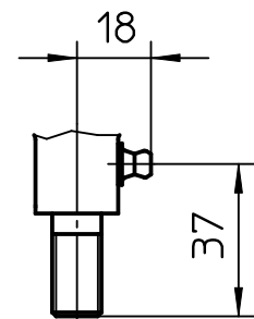
Detail X M 1:2,5
