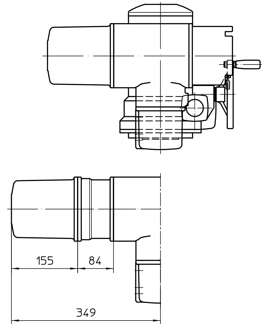
Ausführung mit therm. Überstromrelais Version with thermal overload relay
