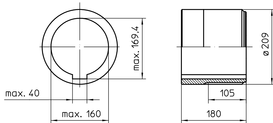
Kupplung
