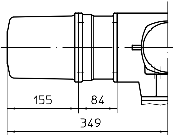
Ausführung mit therm. Überstromrelais
