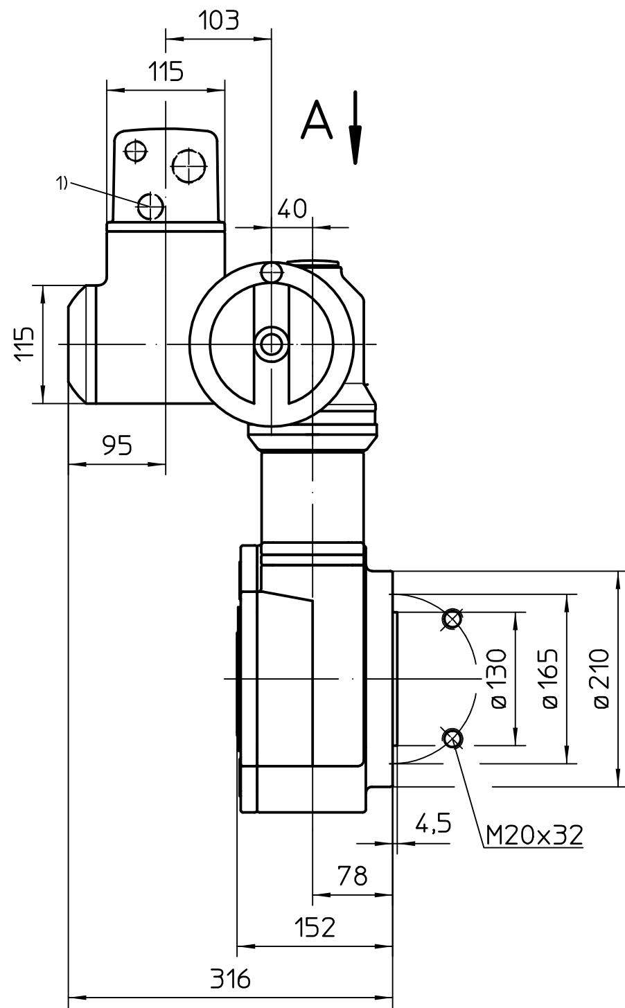
Ansicht A
