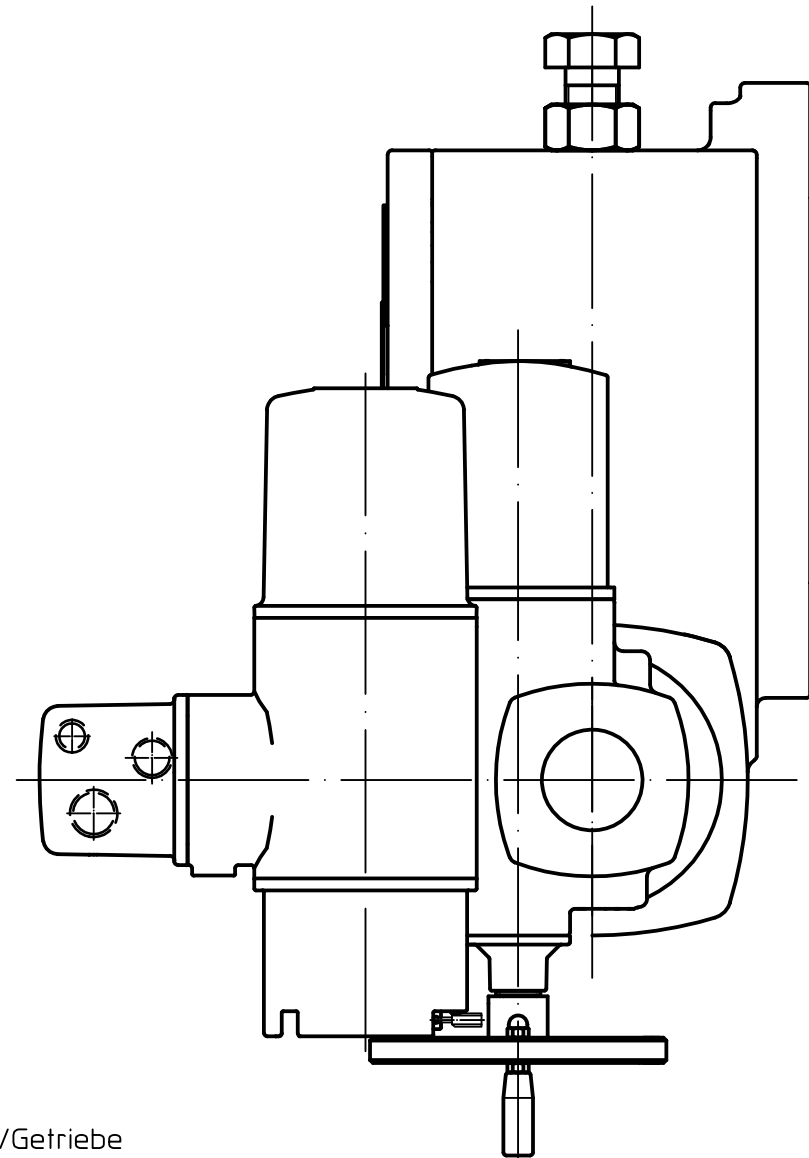
Ansicht A
