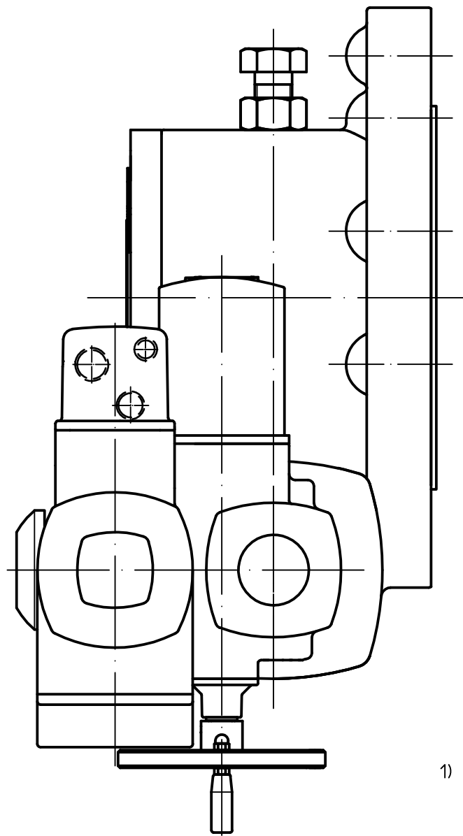
Ansicht A
