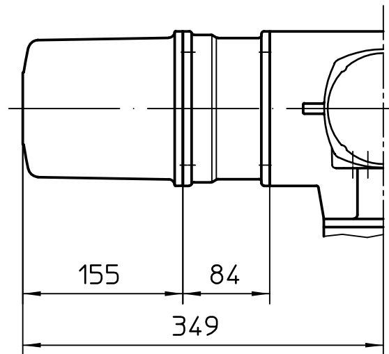
Version avec relais de surcharge therm.
