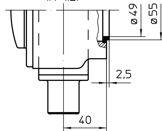
Option Y (M 1:2)
