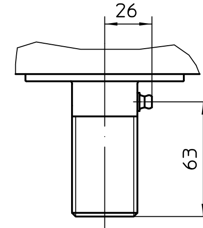
Détail X M 1:2
