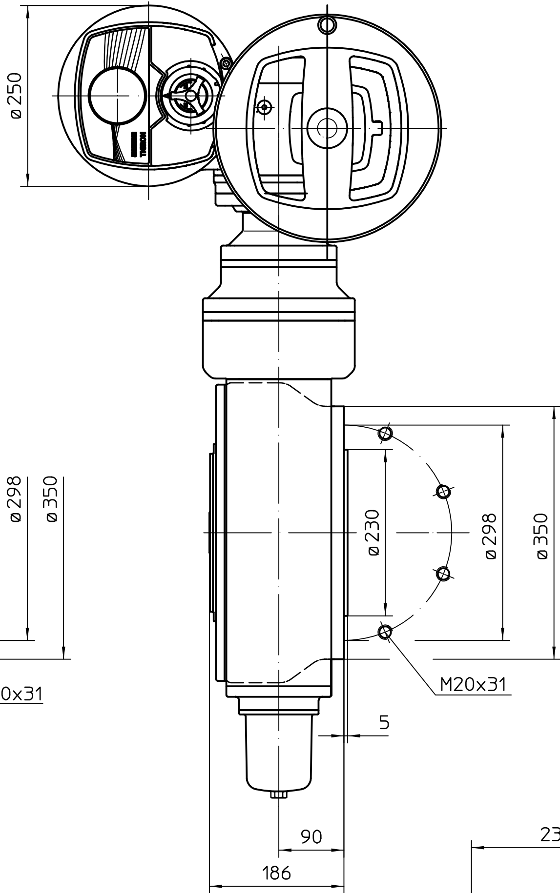
Vue A
