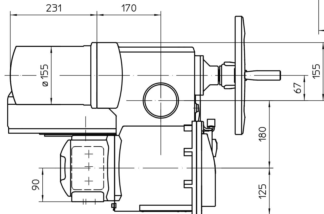
Vue A
