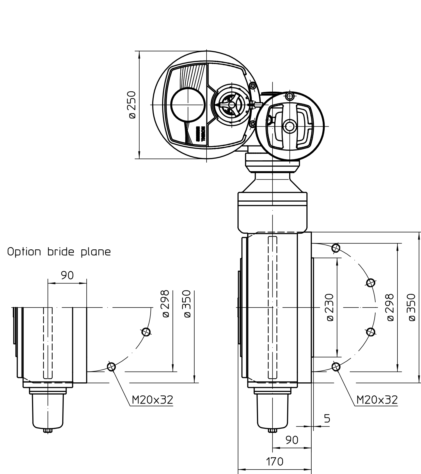
Vue A
